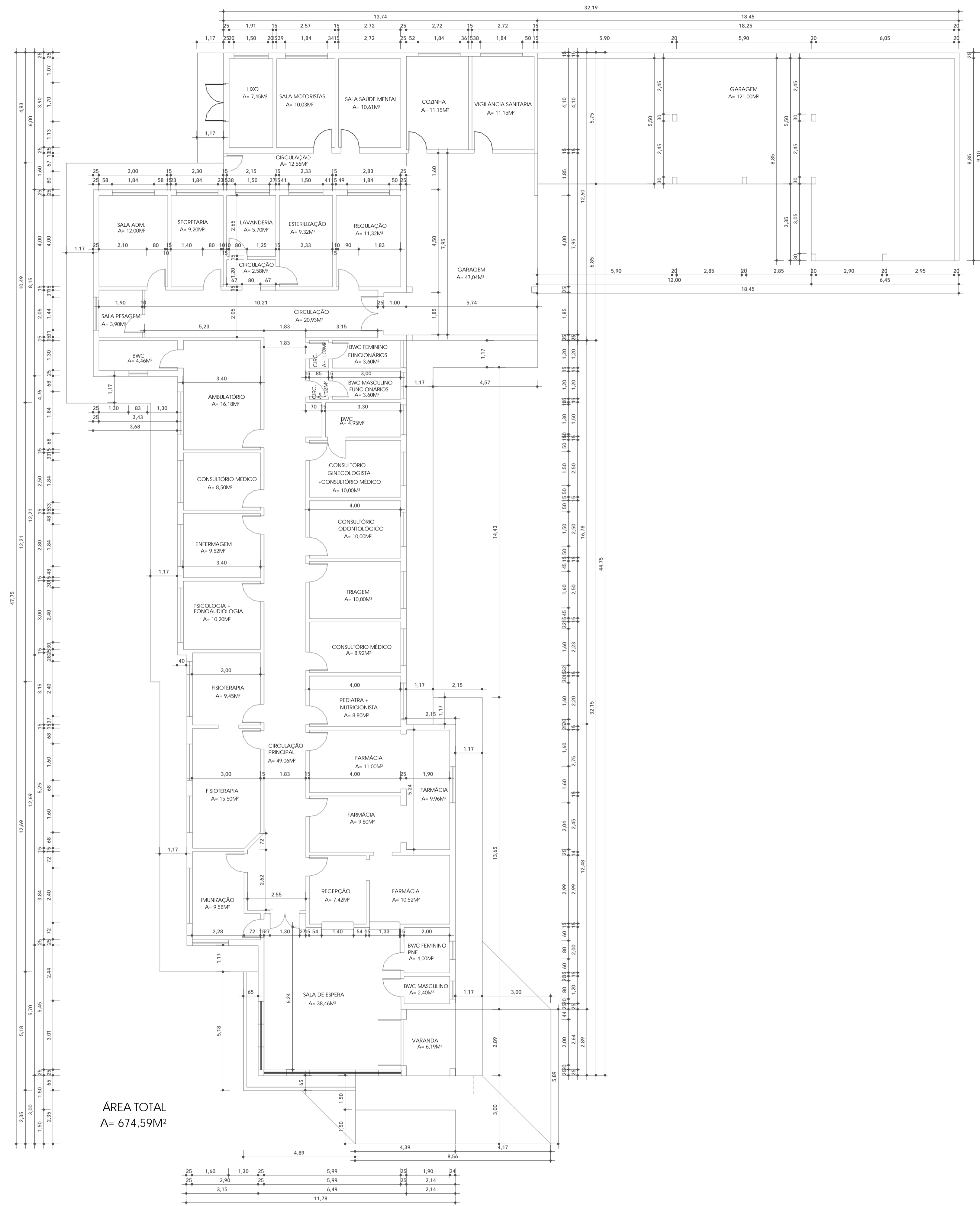
PLANTA BAIXA TÉCNICA ESC: 1 : 100
